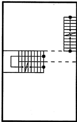
直通樓梯例(一) 虛線範圍表示樓梯間
